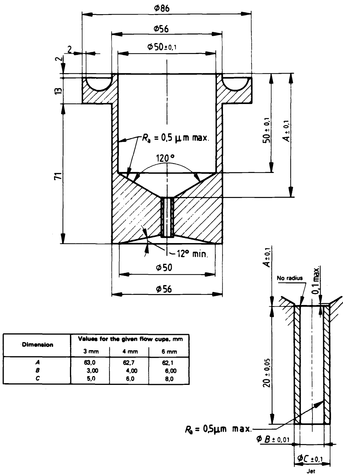
FIG. 1—Flow cup (ISO 2431).
